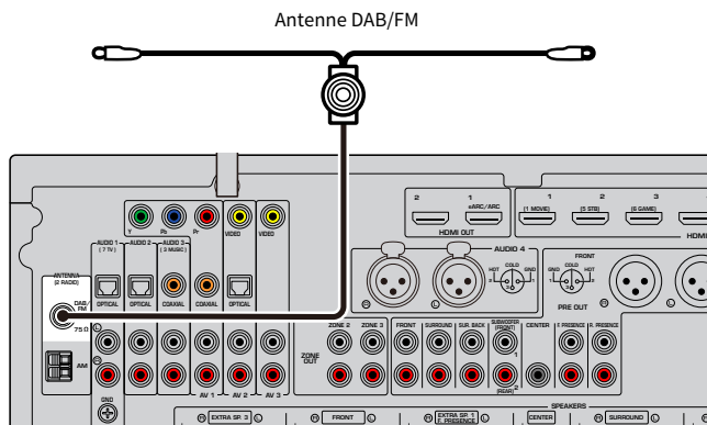
L'unité (arrière)
