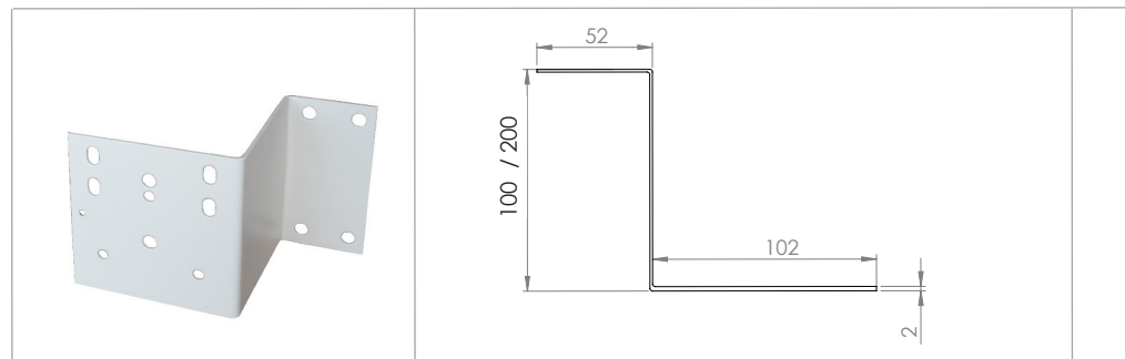
Schéma patte 10 et 20 cm
